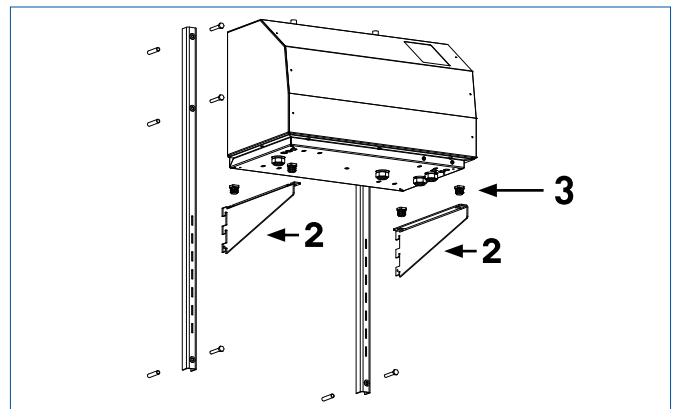
Bevestig de warmtepomp op de muurframe
