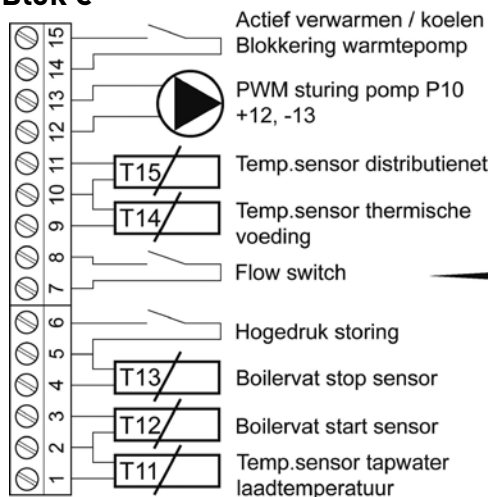
Elektrisch aansluitschema
