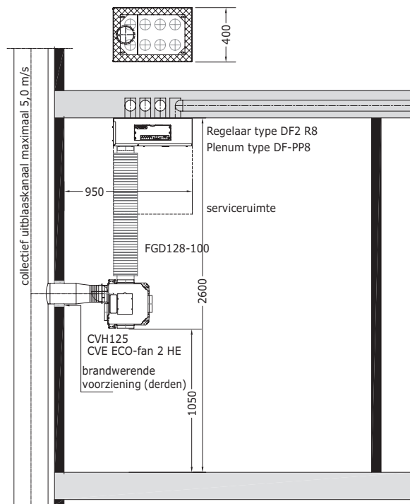
VOORBEELD OPSTELLINGSRUIMTE PLENUM TYPE DF-PP8 - instorten van kanalen \varnothing 80 mm is mogelijk
