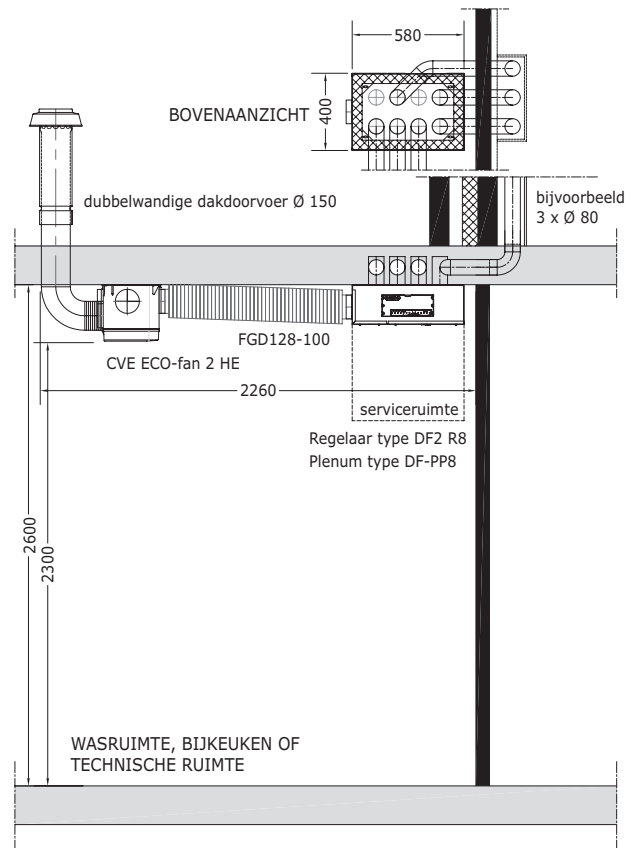
VOORBEELD OPSTELLINGSRUIMTE PLENUM TYPE DF-PP8 - instorten van kanalen \varnothing 80 mm is mogelijk
