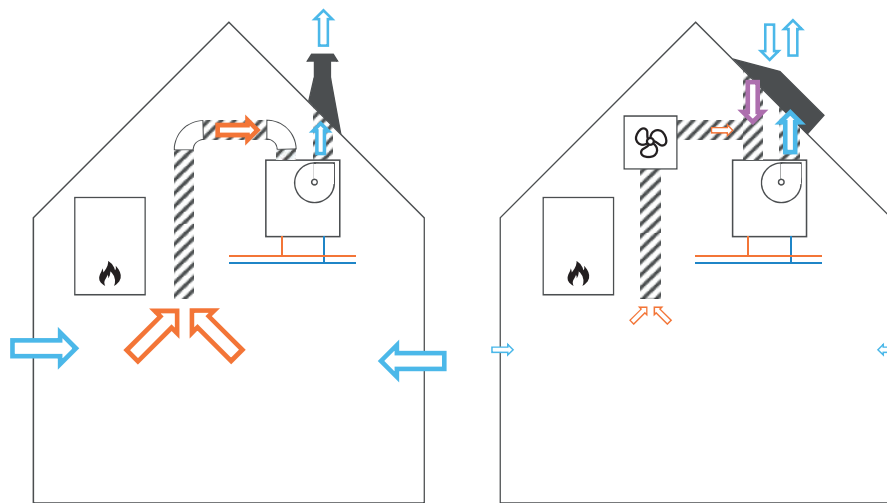
Ventilatorretourlucht warmtepomp
